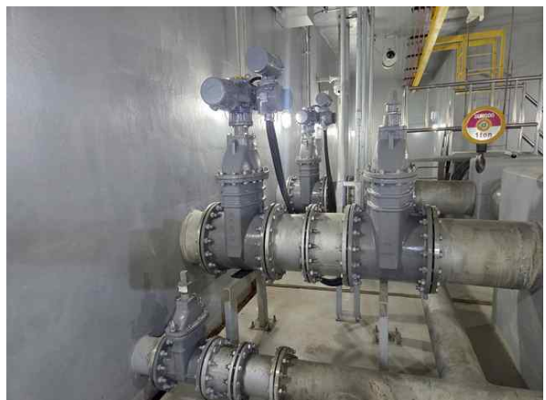
<유출밸브실 유출조절밸브 상태양호>
