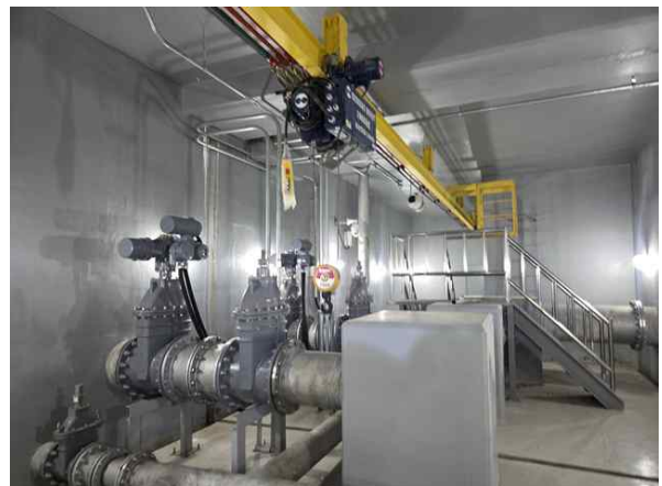
<유출밸브실(지하2층) 전경>
